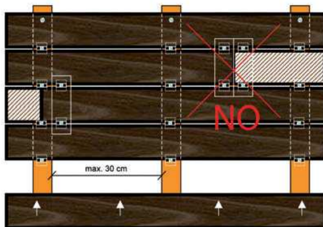
SCHEMA DI MONTAGGIO PAVIMENTO DA ESTERNO IN LISTONI (con impiego di piastrine metalliche)
